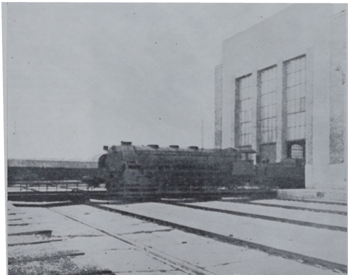
Fachada principal y carro transbordador del nuevo Taller de Montaje, de Valladolid.
