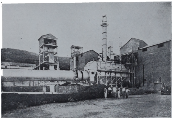
Fábrica de Cemento en Sacedón. Producción: 50,000 toneladas año. Instalada exclusivamente para la construcción de estas obras. Montada en los años 1946, al 1948, y funcionando, normalmente, a partir de Octubre de 1948.
