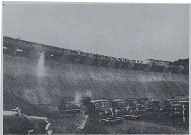
ARROYO (SANTANDER).—Una vista del pantano del Ebro, inaugurado por S.E. el Jefe del Estado. (FOTO CAMPUSA).
