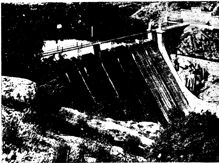
El Gobierno Español acaba de terminar las obras de embalse y presa sobre el río Aulencia, que proporcionará agua a los pueblos de Brunete, Villanueva de Brunete, Villanueva de la Cañada y Quijorna.
