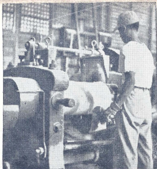
La máquina a donde se pasan las piezas de goma antes de ser cortadas las suelas para los zapatos.
